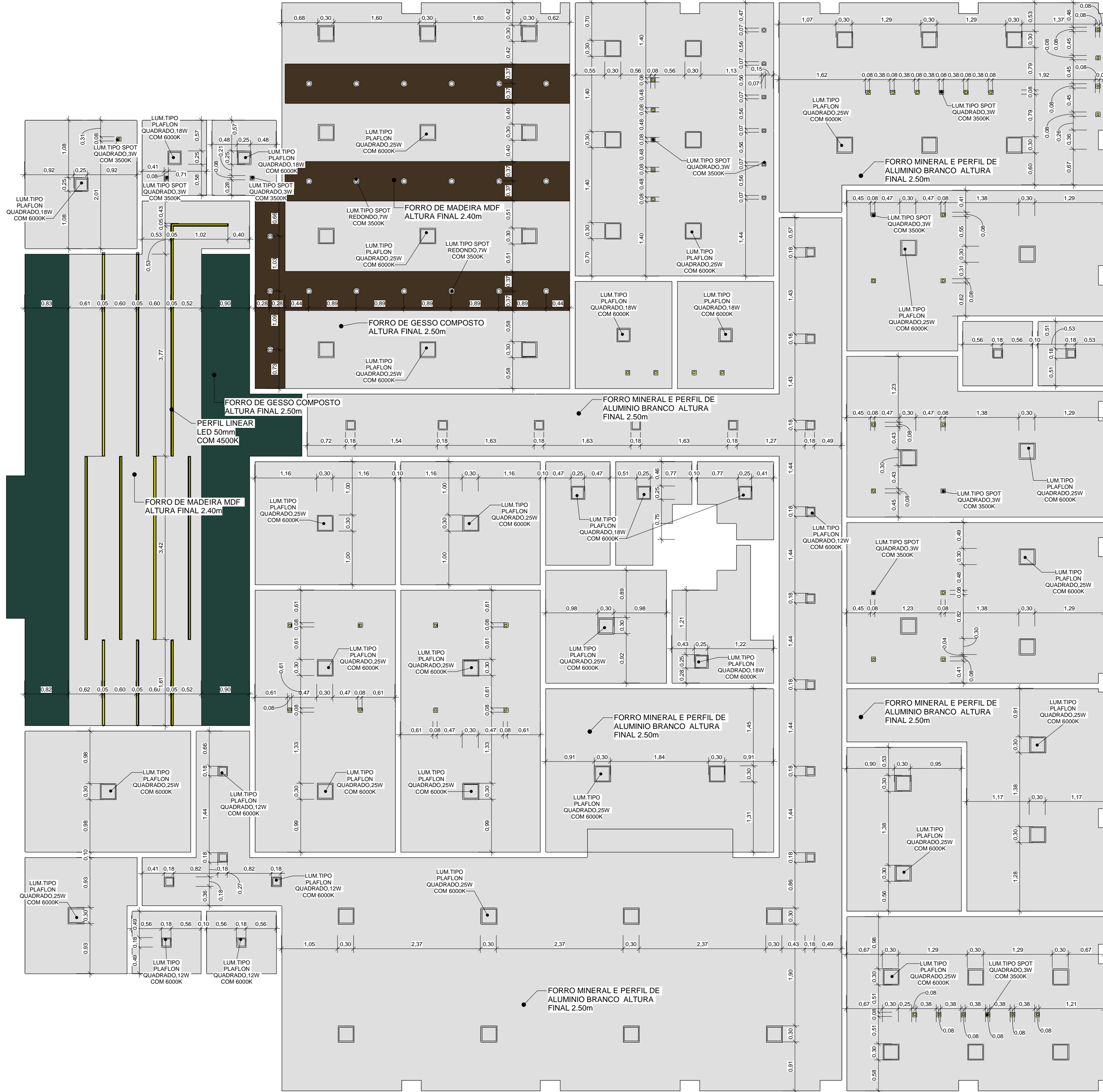
1 PLANTA DE FORRO E ILUMINAÇÃO ESCALA 1 : 50
